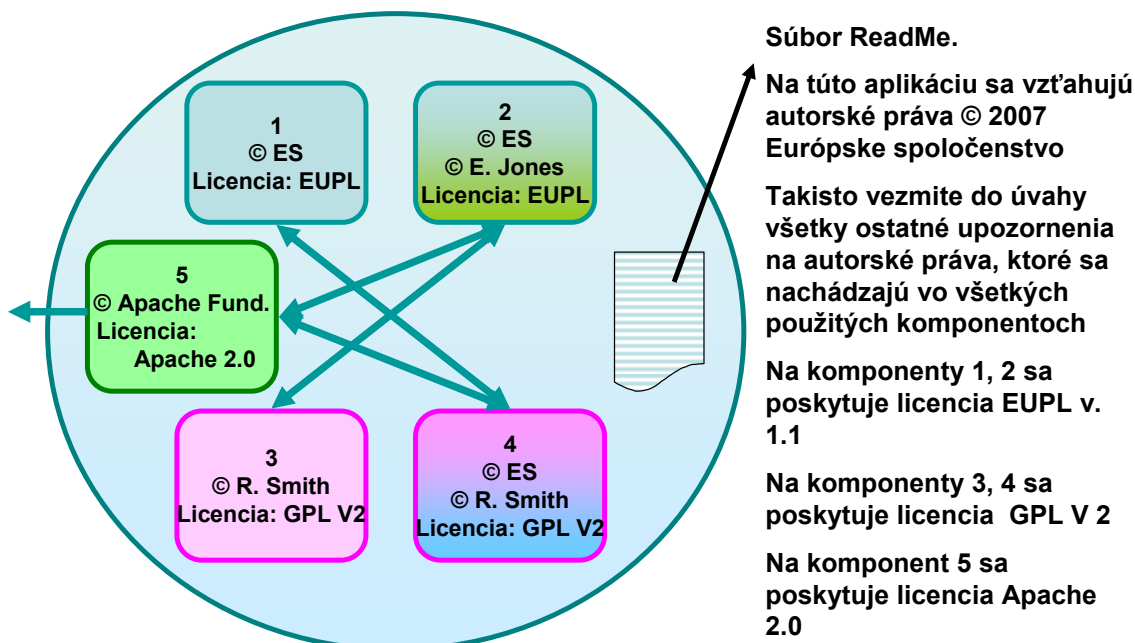
Obr. 4: Integrácia rozličných komponentov
