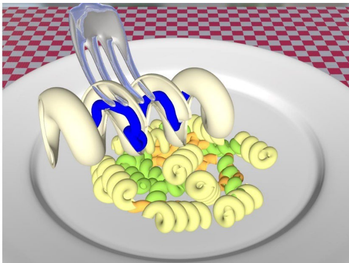
Obr 1: Umelecký pohľad na zauzlenú DNA geometricky obmedzenú v špirálovom nano-kanáli. Uzly na DNA (chirálné superštruktúry) sa vyskytujú prirodzene, ale môžu byť vnesené molekulovou manipuláciou pomocou mechanických pinziet. Špirálové nano-kanály môžu byť pripravené vo forme gélov, živíc alebo molekulových sít a môžu byť použité pre nano-zariadenia v vznikajúcej oblasti chirálnej nanotechnológie (Rusková R. https://doi.org/10.3390/polym13213726 )
